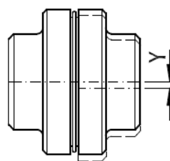
Desalinhamento radial
